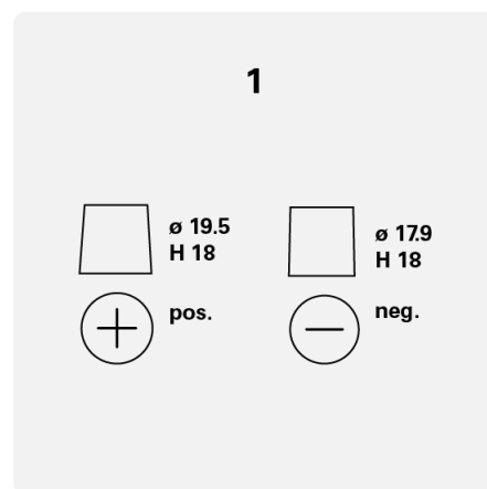
Soort klemmen
